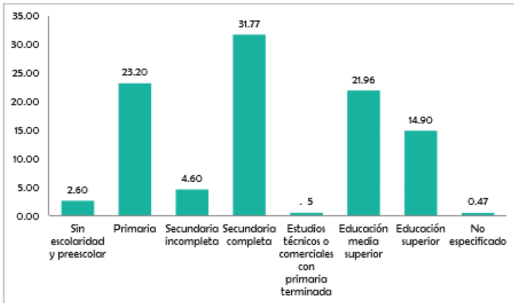
Gráfica 4. Población Económicamente Activa ocupada por escolaridad.
